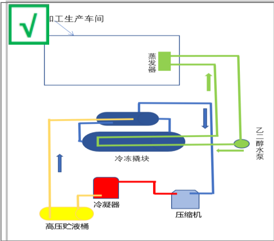
乙二醇空调间接制冷系统
