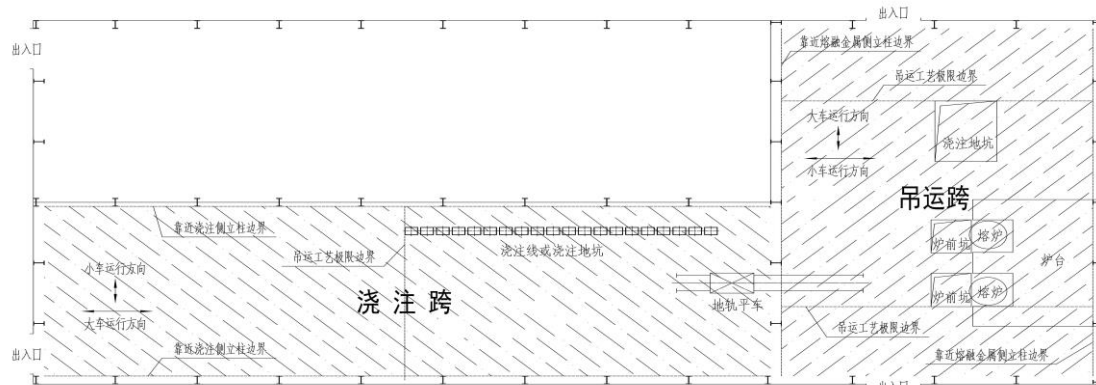
图 7 吊运跨、浇注跨示意图
