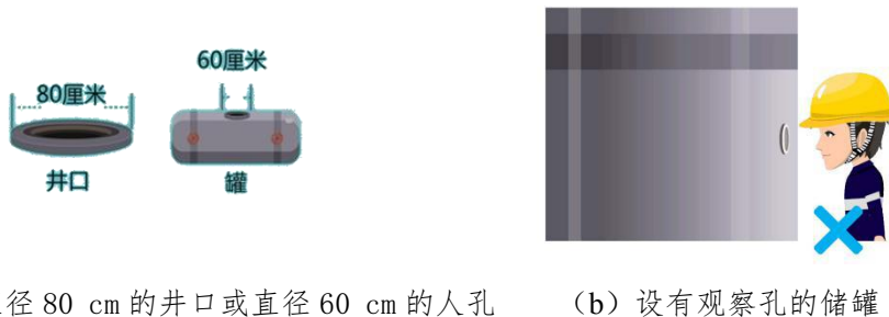
图 1-2 有限空间进出口受限但人员可以进入
